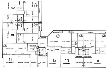
2e VERDIEPING 1100
