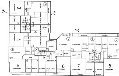
1e VERDIEPING 1100
